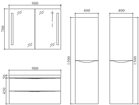
ANCONA-N-900 Basin#28 0900 10(W900mm*D480mm*H140mm) Cabinet#17 0900 65.GH(W900mm*D480mm*H800mm) Storage-L#47 1500 42.JB-T2(W400mm*D300mm*H1500mm) Storage-R#47 1500 43.JB-T2(W400mm*D300mm*H1500mm) Mirror#34 0900 40(W900mm*D126mm*H700mm)
