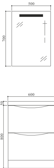
ANCONA-N-SF-600 Basin#28 0600 20(W600mm*D420mm*H140mm) Cabinet#17 0600 97.GB(W600mm*D420mm*H800mm) Mirror#34 0500 40(W500mm*D126mm*H700mm)
